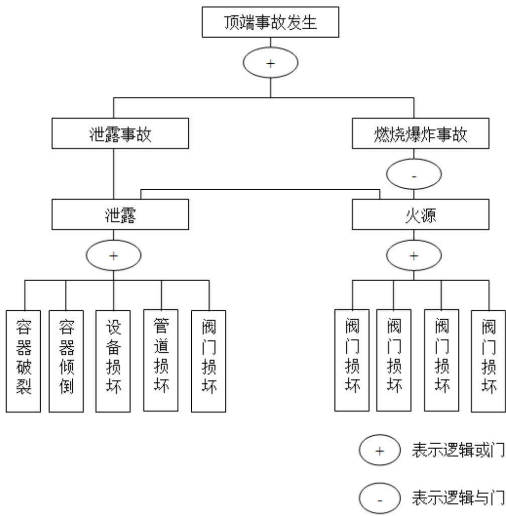
图 8.3-1、顶端事故与基本事件关联图
