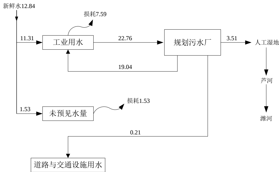
图 7.2-1、园区水平衡图（万m³/d）
