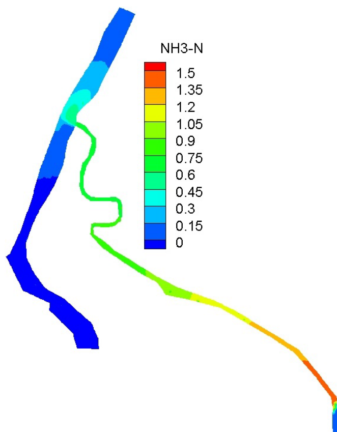
图 7.2-9、规划污水处理厂运行后NH 3 -N浓度分布图（枯水期水文条件）
