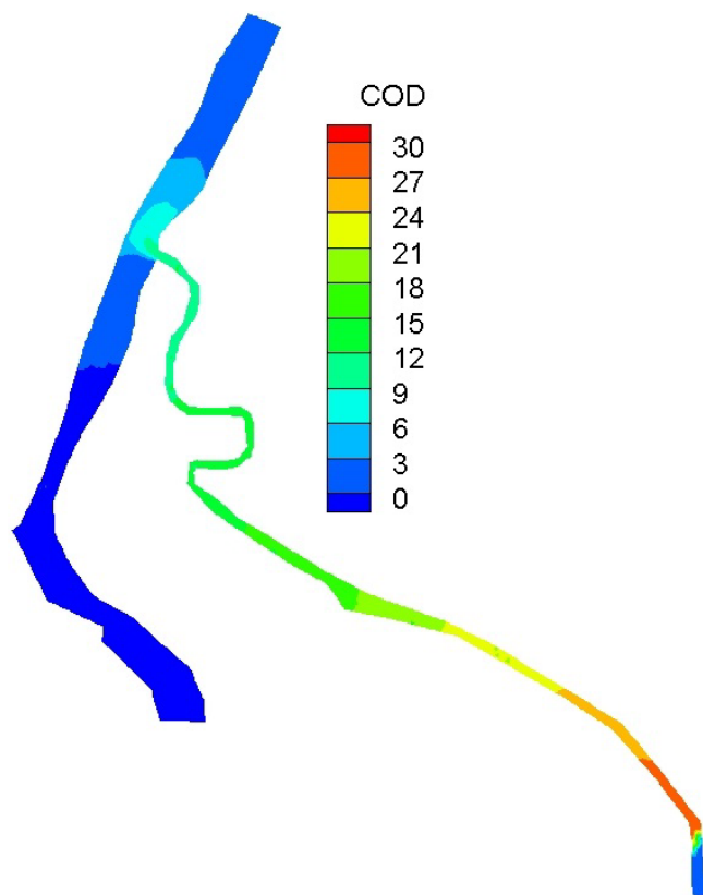
图 7.2-8、规划污水处理厂运行后 COD 浓度分布图（枯水期水文条件）
