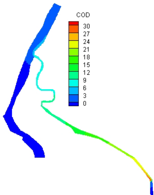
图 7.2-4、规划污水处理厂运行后 COD 浓度分布图（丰水期水文条件）
