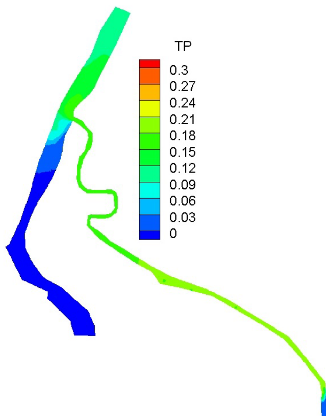
图 7.2-11、诸城污水处理厂运行后 TP 浓度分布图（枯水期水文条件）
