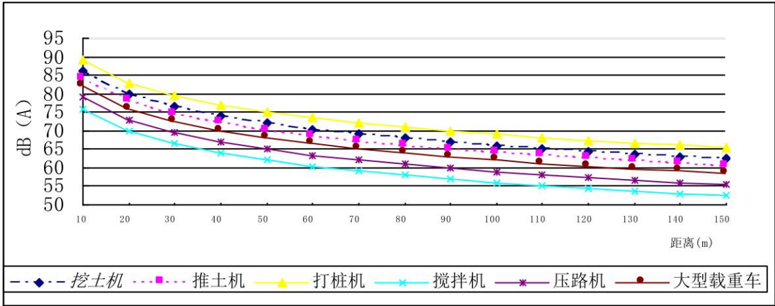
图 7.4-1、单台设备不同距离处噪声强度
