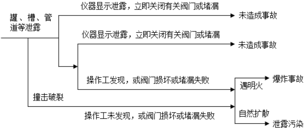
图 8.3-2、事件树示意图
