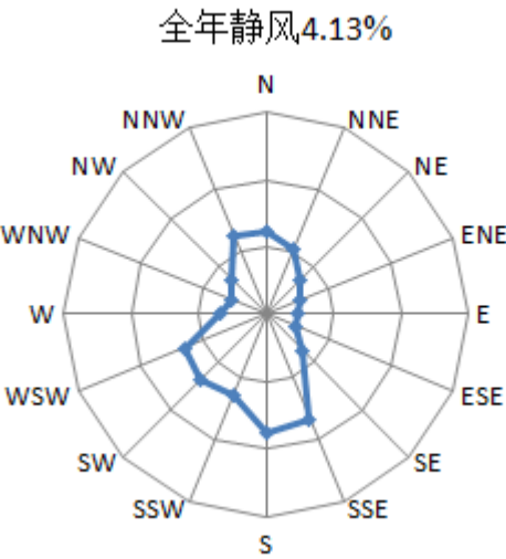
图 7.1-1、诸城近 20 年（1988～2007 年）风向频率玫瑰图
