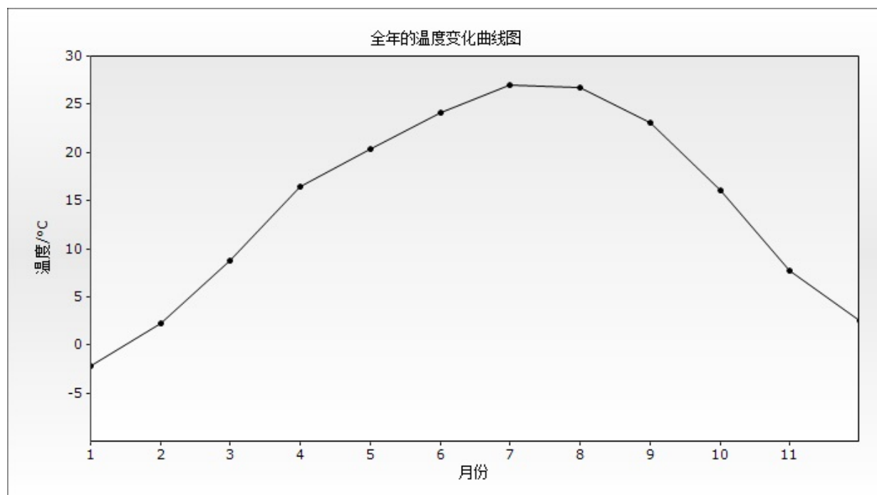
图 7.1-5、2016 年诸城年平均温度月变化曲线
