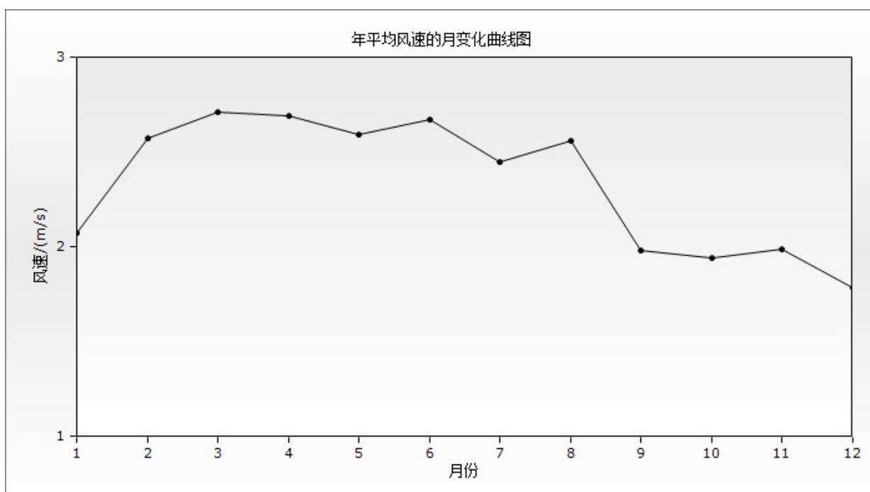
图 7.1-2、诸城年平均风速月变化曲线
