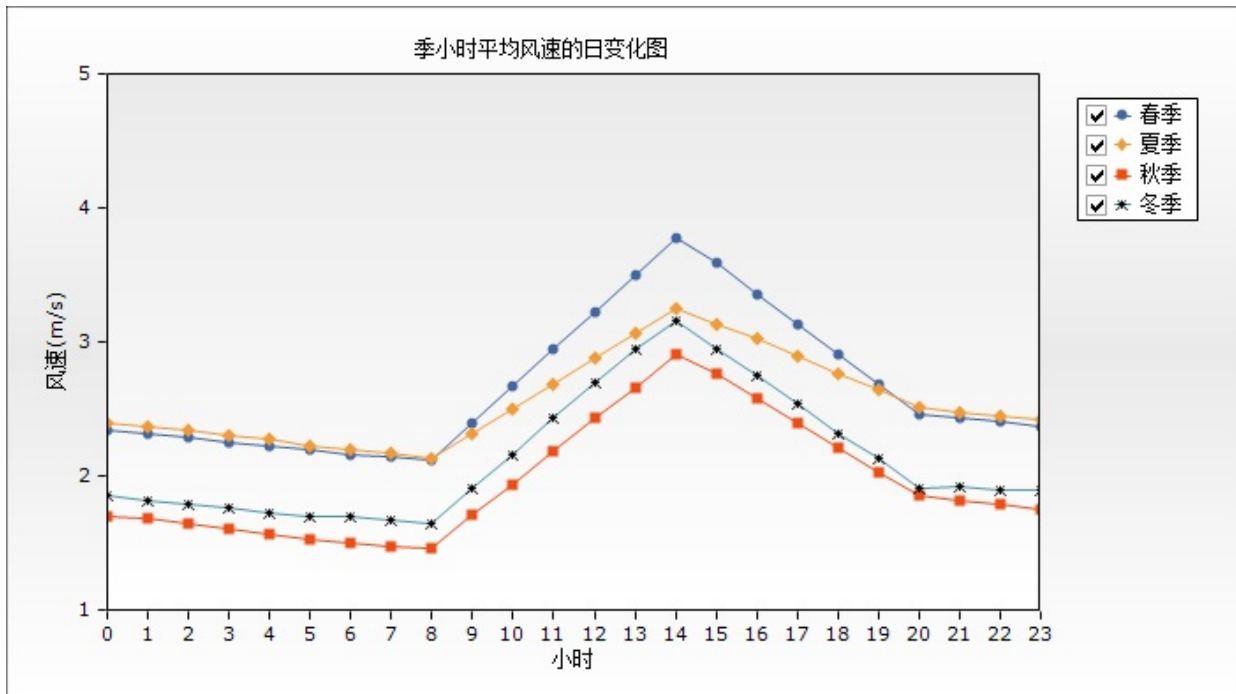
图 7.1-3、2016 年诸城季小时平均风速日变化曲线
